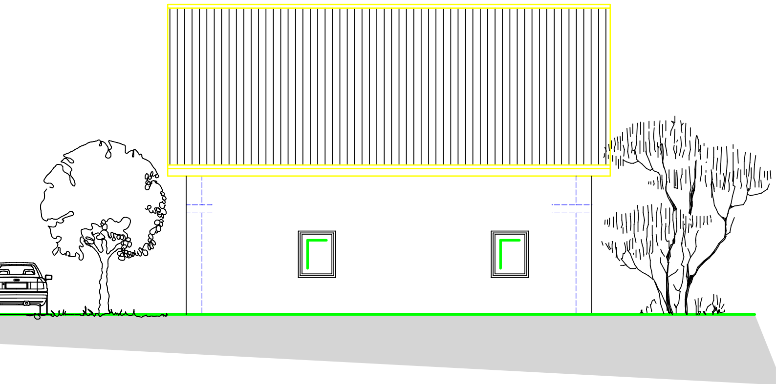
nordansicht
