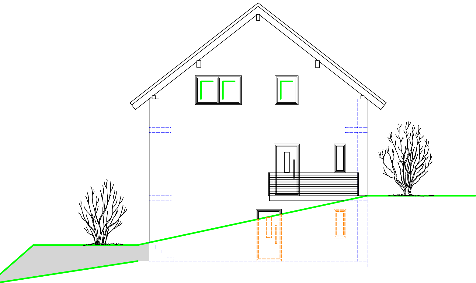
ostansicht
