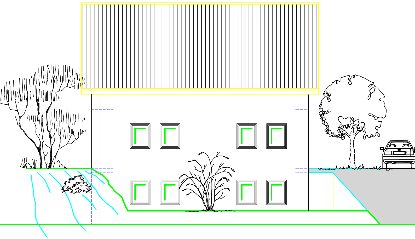
südansicht
