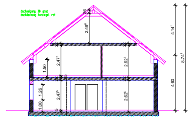
schnitt
