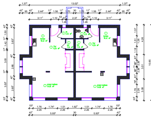
erdgeschoss
